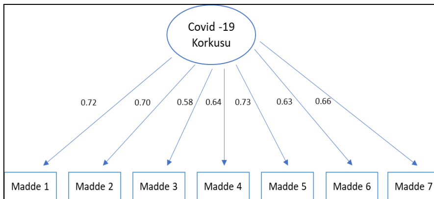
Şekil 1. Covid -19 Korkusu Ölçeği'nin Doğrulayıcı Faktör Analizi (DFA) Sonuçları
