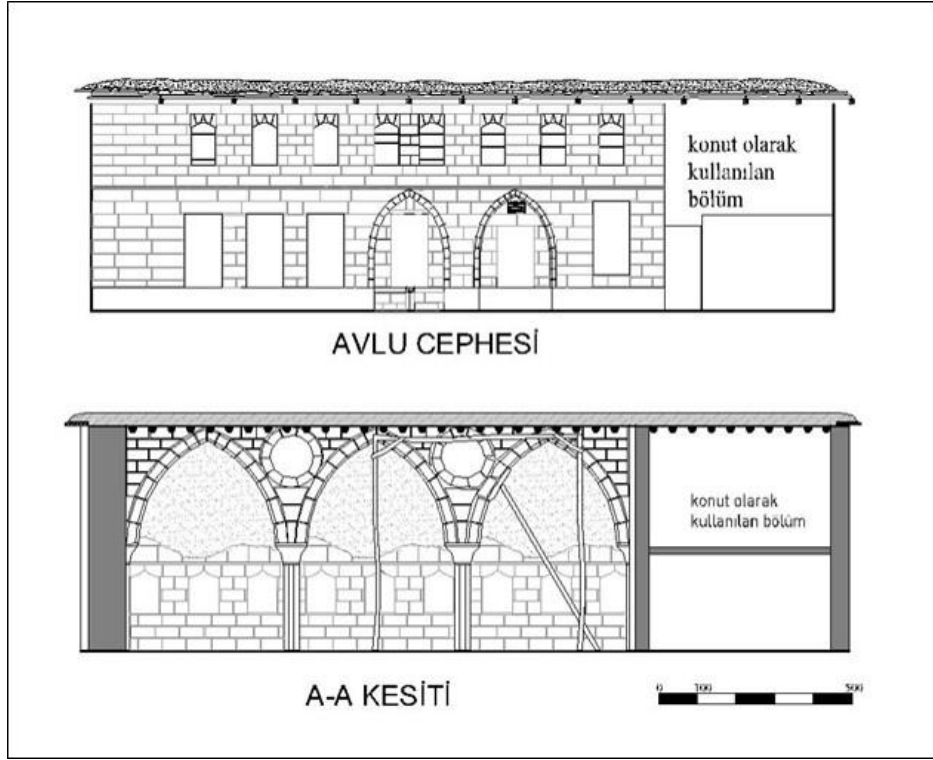
Şekil 5. Sinagog Kesit ve Cephe Krokisi (Kakdaş Ateş; Payaşı Oğuz, 2019)
