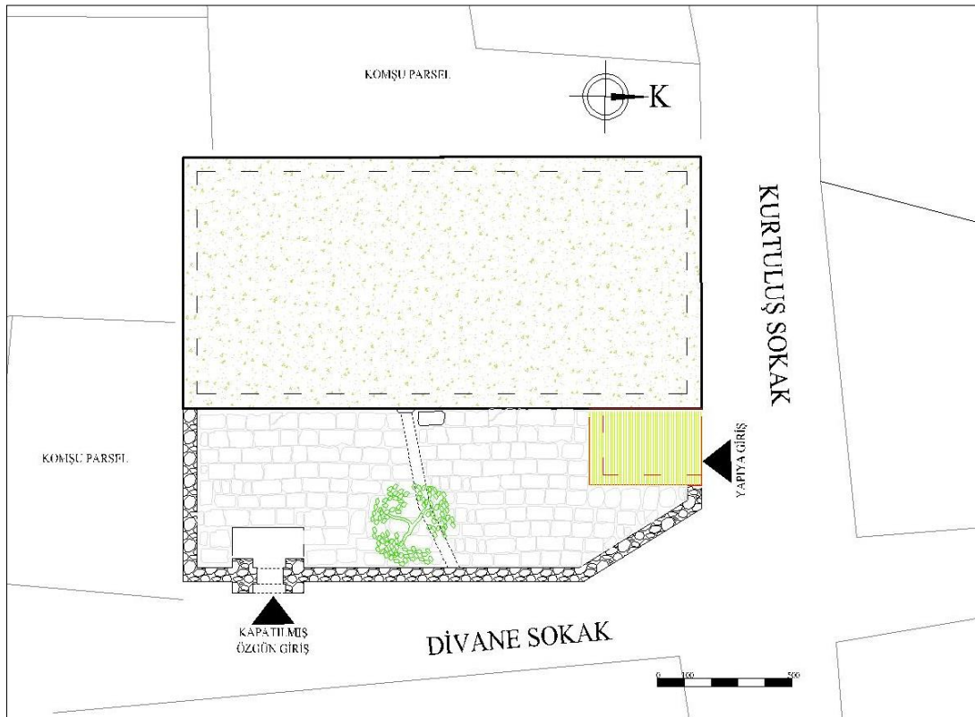
Şekil 3. Çermik Sinagogu Vaziyet Planı (Kakdaş Ateş; Payaslı Oğuz, 2019)
